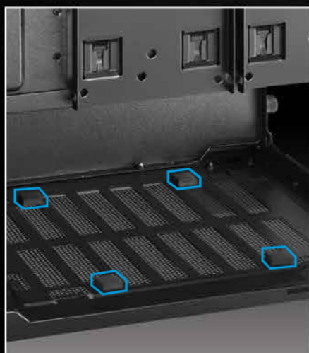
Entkoppelte Netzteilmontage
