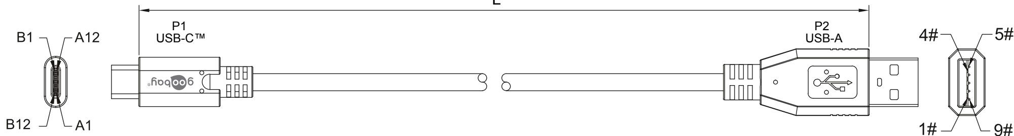
Anschlussdiagramm / Wiring diagram
