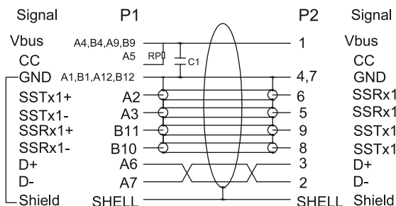
Anschlussdiagramm / Wiring diagram
