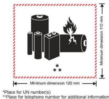
图 4: 锂电池标记
