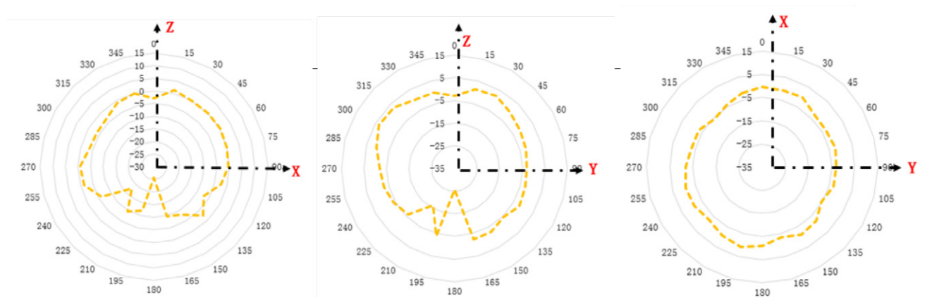
Abbildung 3: BLE-Abstrahlmuster
